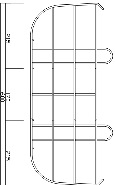
後面 立面図 1/5
