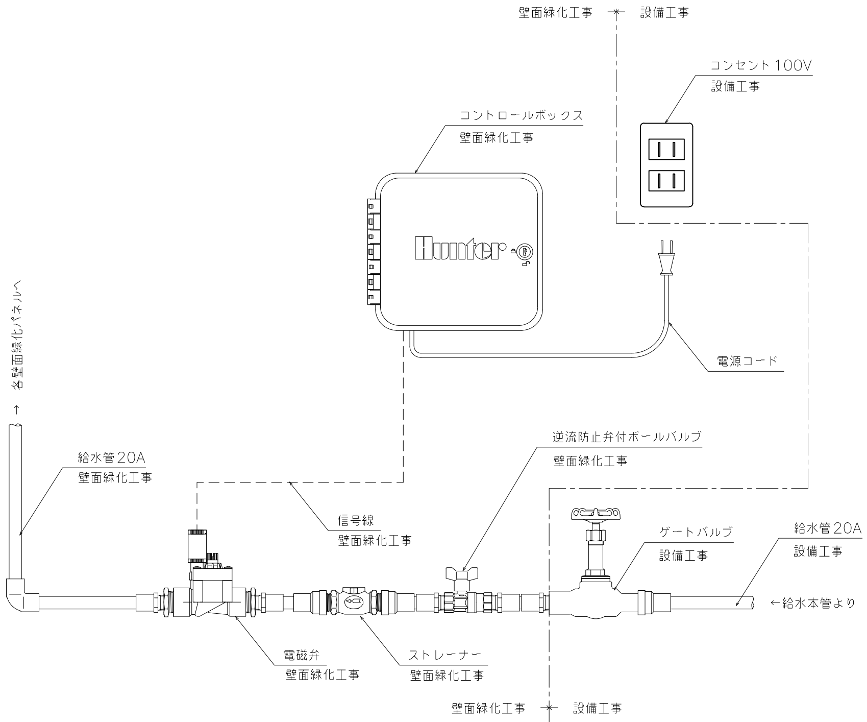
自動灌水装置接続例
