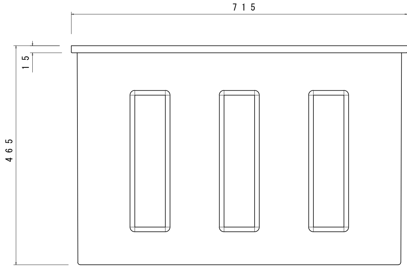
タンク立面図
