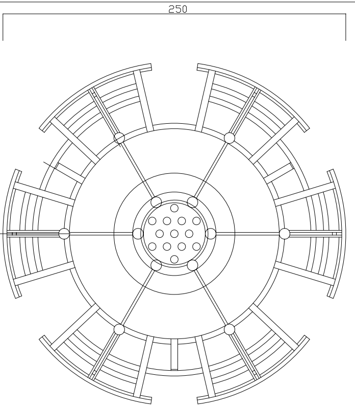
伏図
