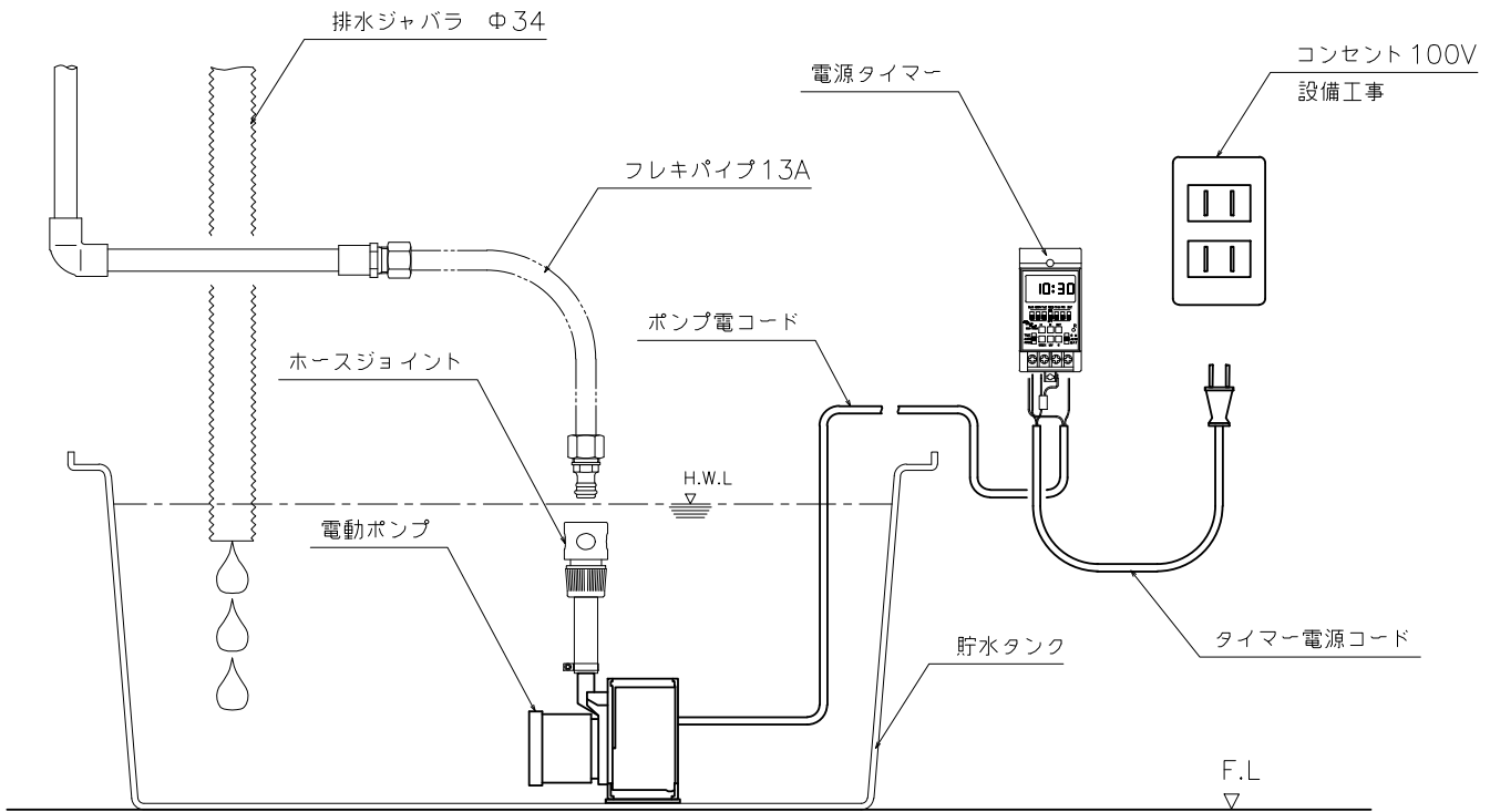
タンク式給排水設備図
