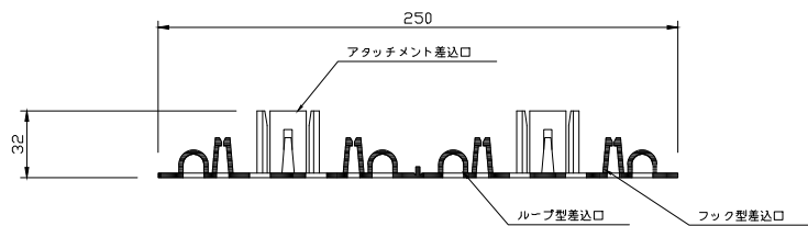
デコプラ基盤側面図
