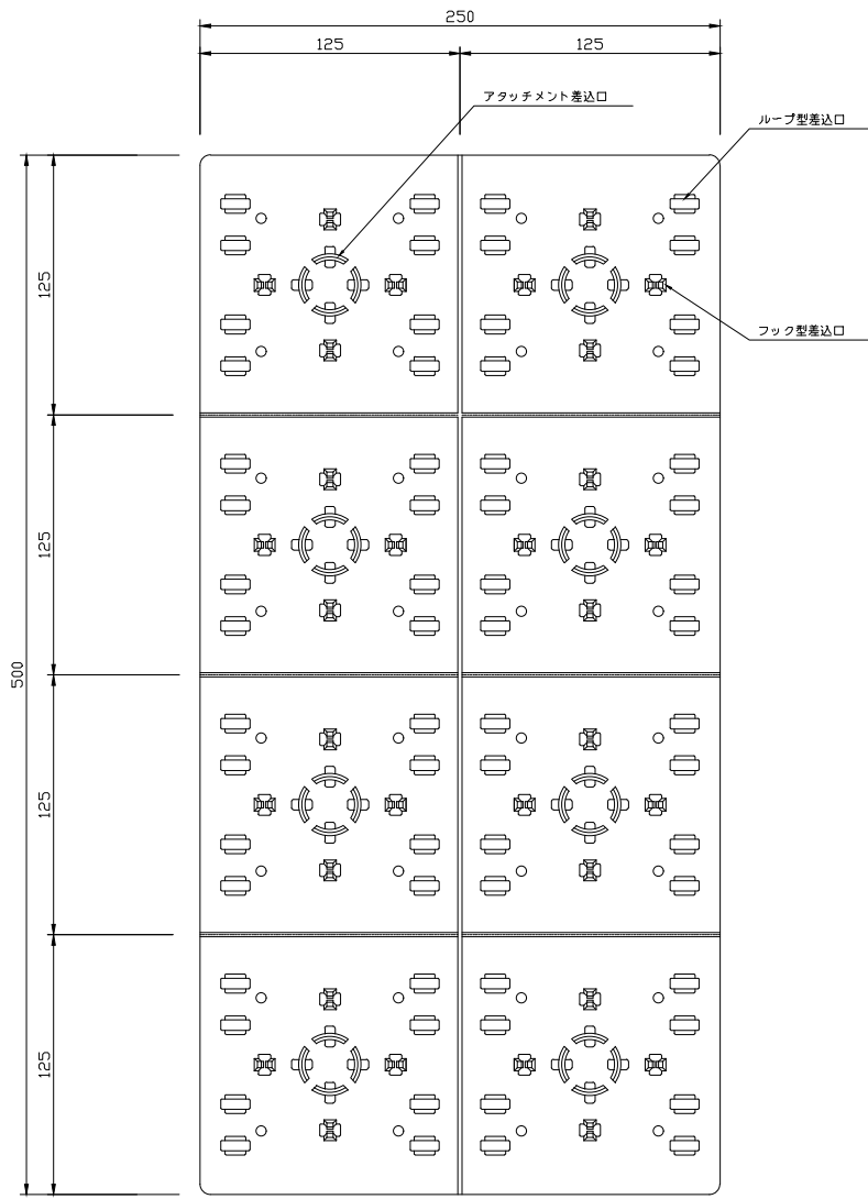
デコプラ基盤平面図
