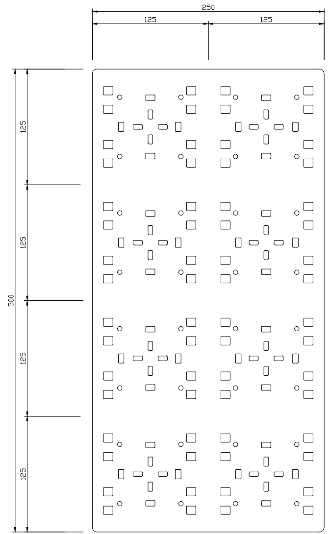
デコプラ基盤背面図
