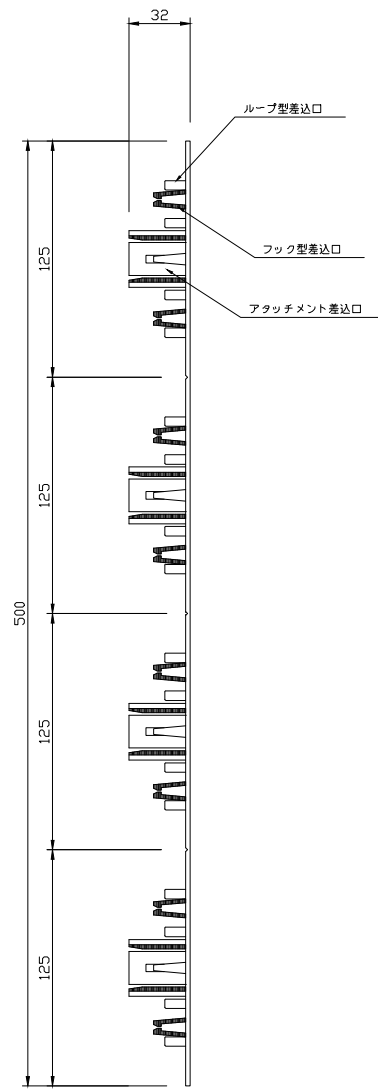
デコプラ基盤立面図
