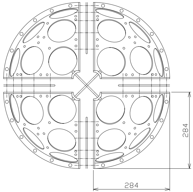
上下 伏図
